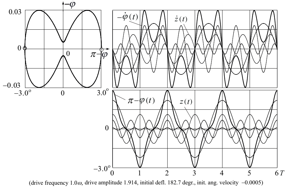
Рис. 7: Флаттер-мода колебаний перевернутого маятника непосредственно над верхней границей динамической стабилизации.
