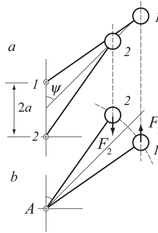
Рис. 1: Поведение маятника с осциллирующей осью в инерциальной (лабораторной) системе отсчета (a) и в системе, связанной с осью (b).
