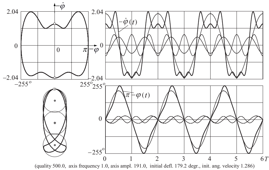
Рис. 9: Колебания большой амплитуды с периодом 2T около перевернутого положения: фазовая траектория (вверху слева), траектория груза маятника в пространстве (внизу слева), графики угловой скорости \dot{\varphi}(t) (вверху справа) и угла отклонения \varphi(t) (внизу справа) вместе с графиками гармонических составляющих.
