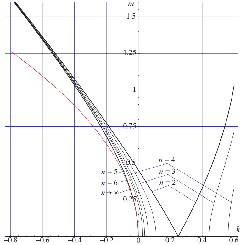
Рис. 3: Относительная амплитуда подвеса m = a/l как функция k = g/(l\omega^2) (квадрата обратной относительной частоты подвеса) в условиях порога субгармонических резонансов нескольких порядков n . Границе области динамической стабилизации перевернутого маятника соответствует левая кривая, обозначенная как n \rightarrow \infty (см. подробности в тексте).
